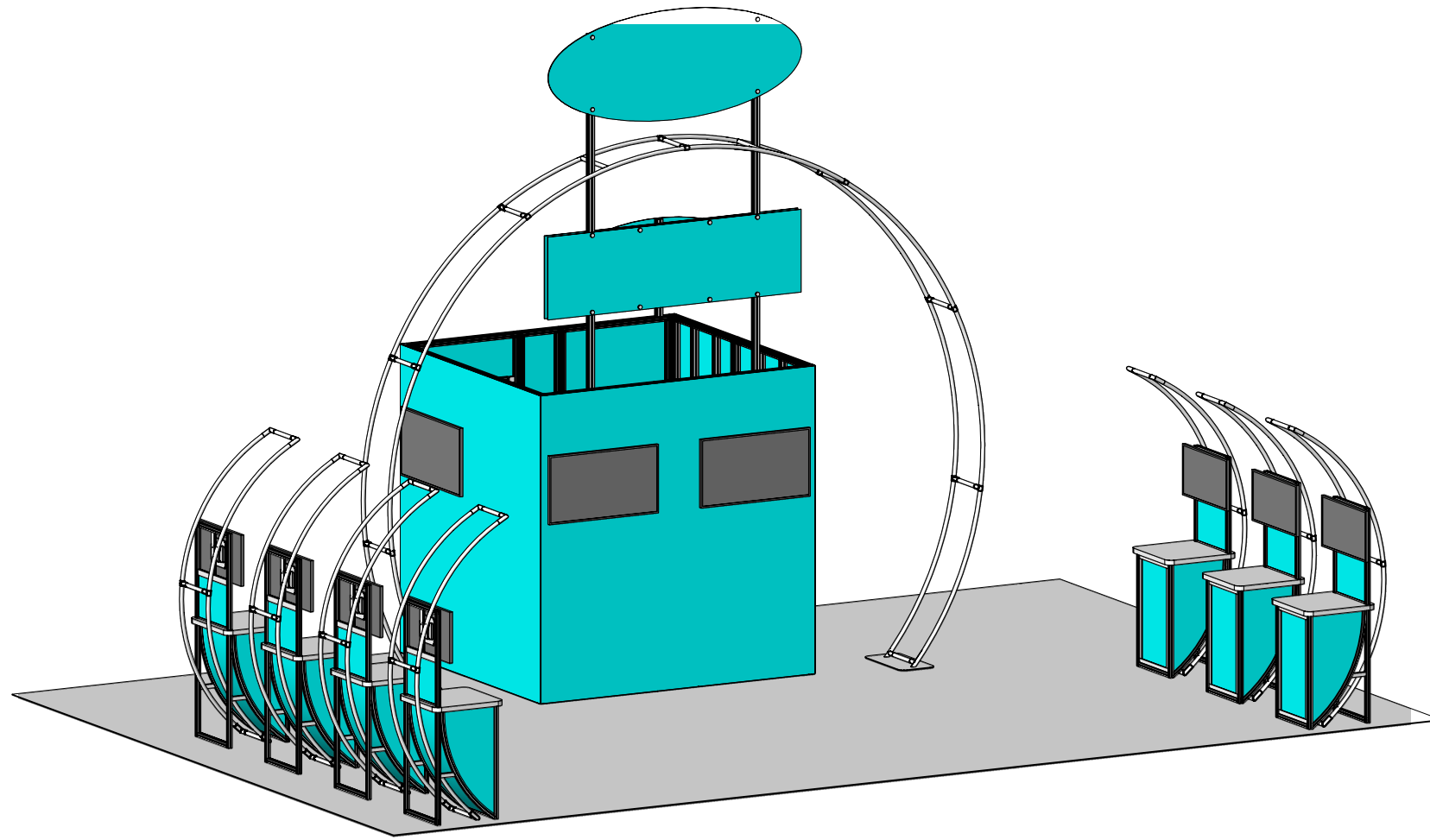
1 ISO Scale: 1:50
