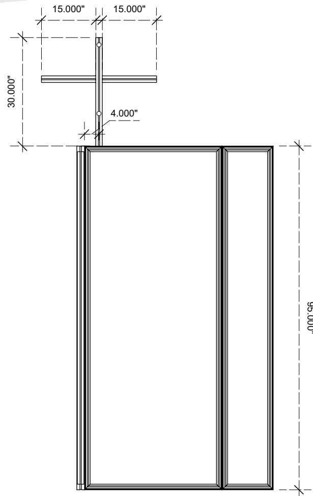
3 Section View Scale: 1:27
